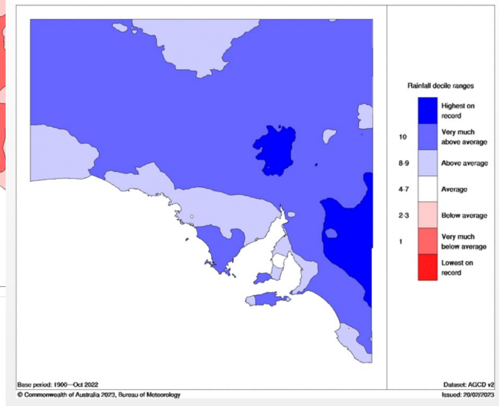
Aug- Oct 2022 deciles
